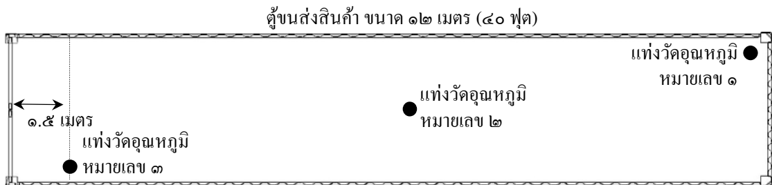
ภาพที่ ๑ ตำแหน่งการวางถังวัดอุณหภูมิผลไม้ภายในตู้ขนส่งสินค้าสำหรับการกำจัดศัตรูพืชด้วยความเย็นในระหว่างขนส่ง
