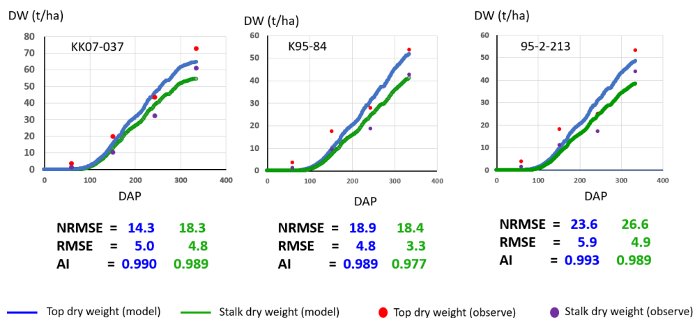
ภาพที่ 2.2.6 ผลการปรับค่าสัมประสิทธิ์ทางพันธุกรรมของอ้อย 3 พันธุ์สำหรับใช้กับแบบจำลอง Canegro
