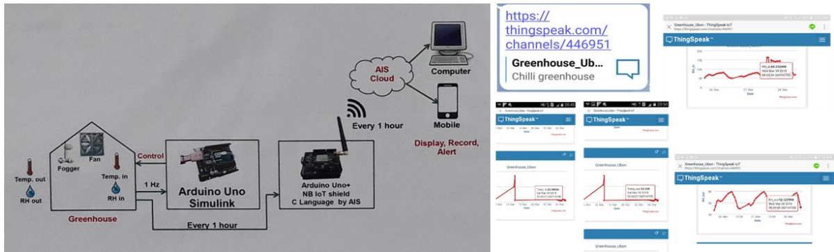
ภาพที่ 19 หลักการอ่านและส่งข้อมูล ผ่านระบบอินเทอร์เน็ตแห่งสรรพสิ่ง (Internet of Things, IoT)
