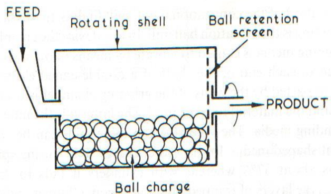
ภาพที่ 6 Ball mill
