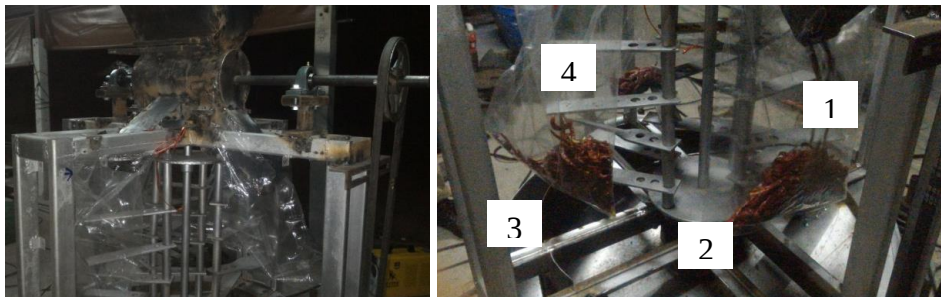
ภาพที่ 23 ทดสอบการป้อนเพื่อปรับการกระจายตัวของพริกที่แต่ละช่องป้อน
