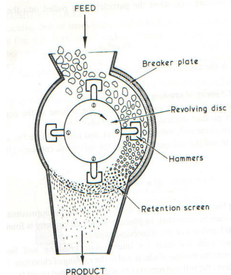
ภาพที่ 2 Hammer mill
