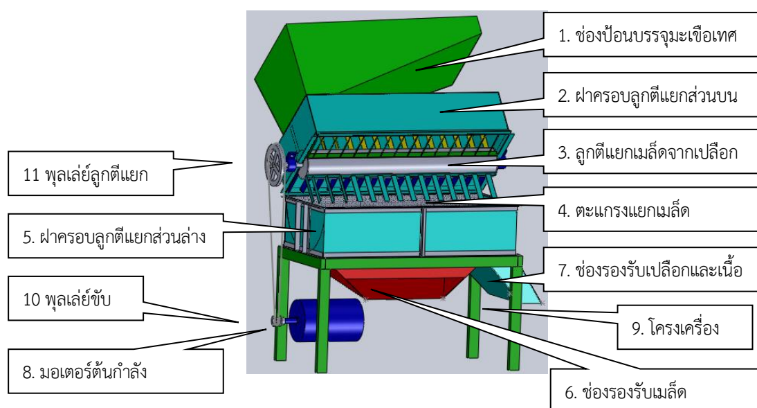
ภาพที่ 37 ภาพร่างการออกแบบเครื่องแยกเมล็ดมะเขือเทศออกจากเปลือก
