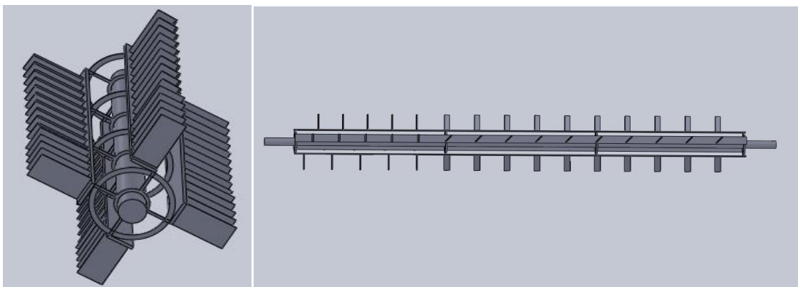
ภาพที่ 38 แสดงลักษณะใบตีแยกเมล็ดมะเขือเทศออกจากเปลือก และแสดงลักษณะการจัดวางใบตี
