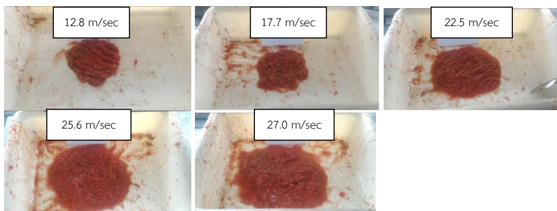
ภาพที่ 42 เมล็ดและเนื้อมะเขือเทศที่ผ่านตะแกรงลงสู่ช่องรับเมล็ด ที่แต่ละความเร็วของการดีแยก
