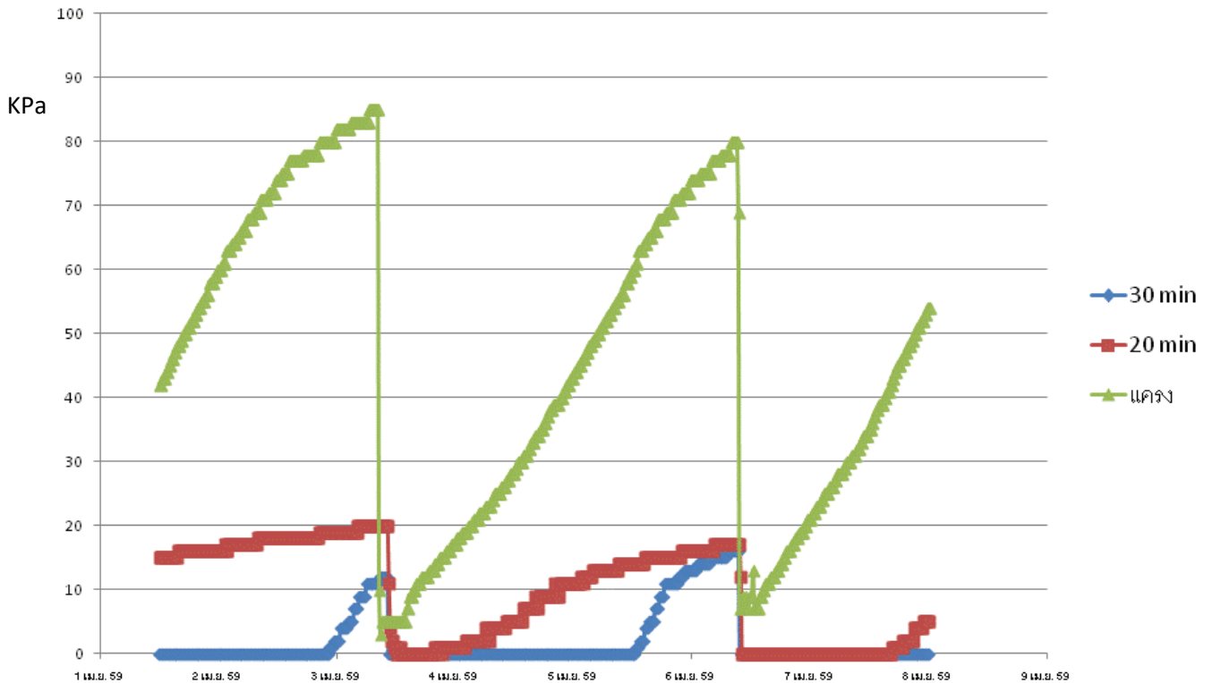
กราฟที่ 1 ค่าแรงดึงน้ำในดิน (KPa) จากการวัดด้วย soil moisture sensor ในช่วงรอบเวรการให้น้ำ
