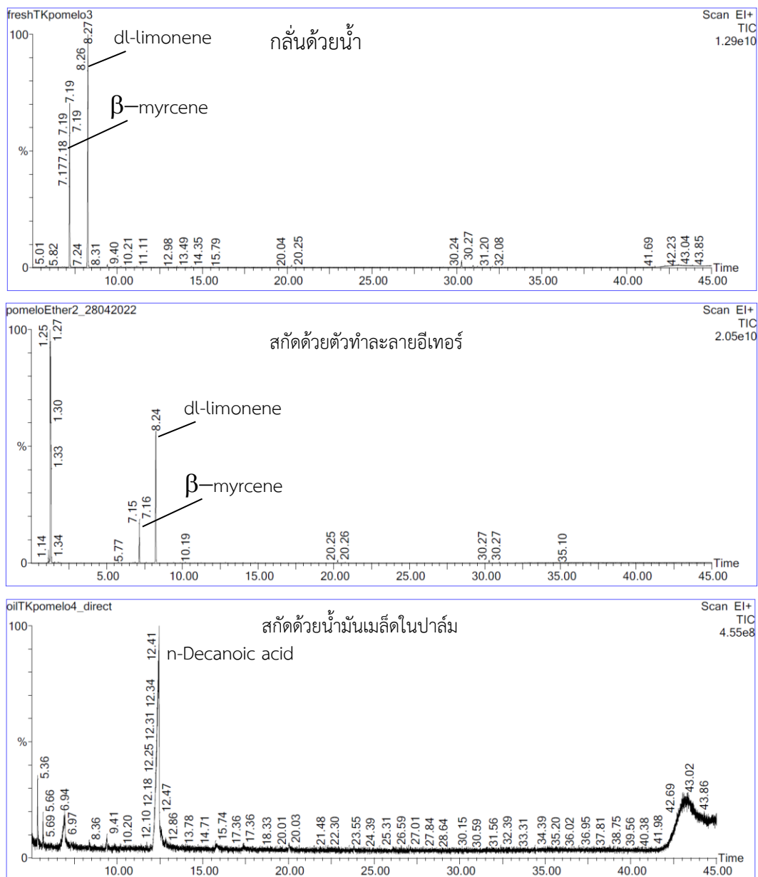
ภาพที่ 5 โครมาโทแกรมน้ำมันหอมจากเปลือกส้มโอทำห่อยที่สกัดด้วยวิธีการต่าง ๆ โดย GC-MS
