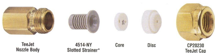
ภาพที่ 1 ชิ้นส่วนต่าง ๆ ของหัวฉีดชนิดใช้แรงดันของเหลว
