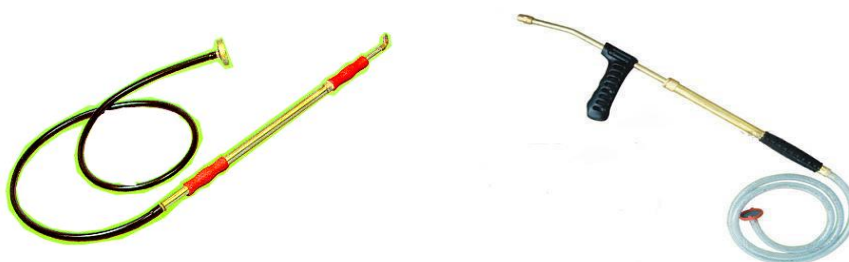
ภาพที่ 8 เครื่องพ่นสารแบบสูบชัก และถังบรรจุสารป้องกันกำจัดศัตรูพืช
