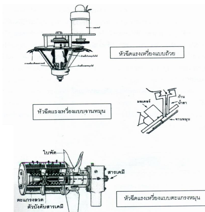
ภาพที่ 7 การเกิดละอองสารของหัวฉีดชนิดใช้แรงเหวี่ยง และตะแกรงหมุน
