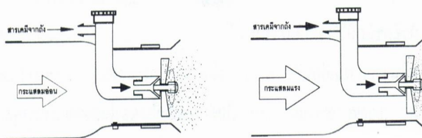
ภาพที่ 6 การเกิดของละอองสารที่ขนาดแตกต่างกันเนื่องจากความเร็วกระแสลมและ อัตราการไหลของของเหลวที่ผ่านลงในกระแสลม
