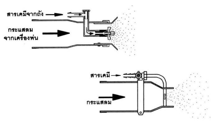
ภาพที่ 5 การเกิดของละอองสารจากหัวฉีดชนิดใช้แรงลม ภาพบนละอองเกิดจากกระแสลม และใบพัดตีของเหลวให้แตก
