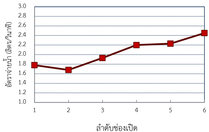
ภาพที่ 5 อัตราการจ่ายน้ำที่จุดต่างๆของชุดให้น้ำด้วยท่อเปิดแบบท่อแข็ง
