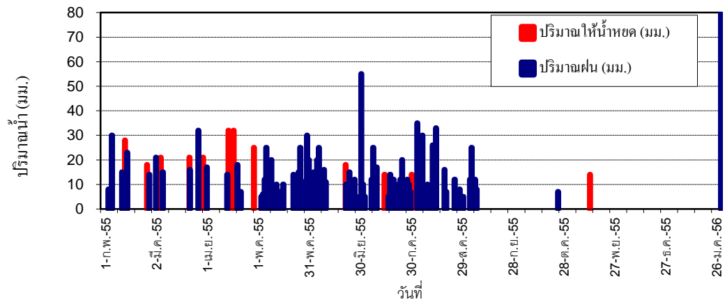
ภาพที่ 6 ปริมาณฝนและปริมาณน้ำที่ให้ได้ด้วยระบบน้ำหยด ที่แปลงทดสอบ จ. สุพรรณบุรี ปี 2555
